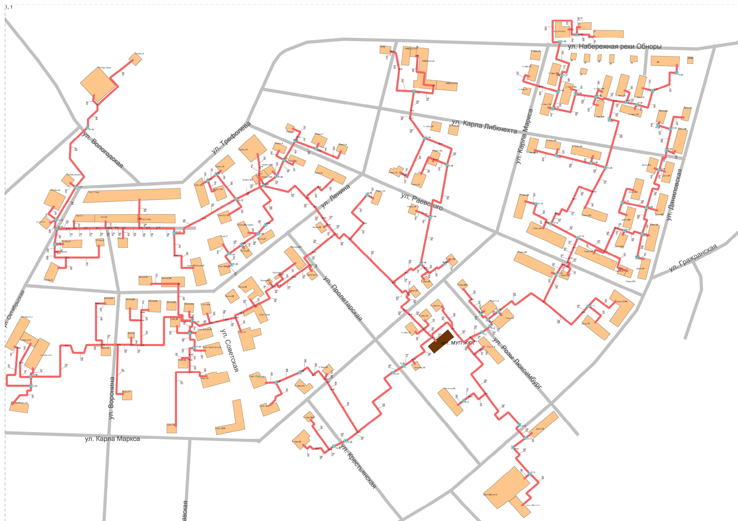
Схема тепловых сетей (отопление) центральной котельной
