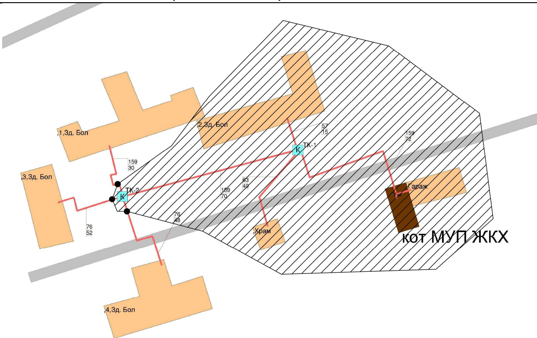
Рис. 6. Зона эффективного теплоснабжения для котельной п. Отрадный
